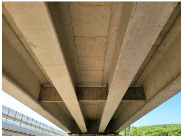
바닥판하면 전경
