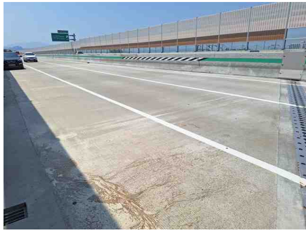
교면포장 전경
