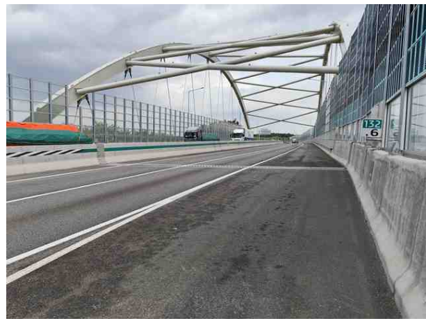
교면포장 전경
